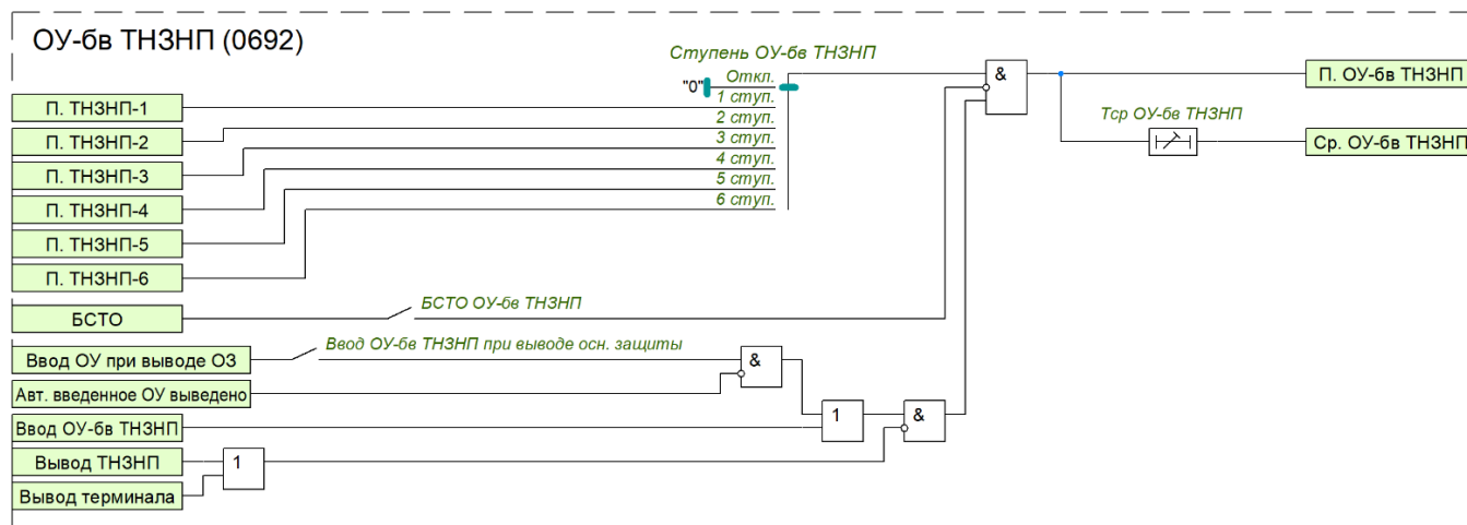
Рисунок 1.23 – Функциональная схема ОУ-6в ТНЗНП
